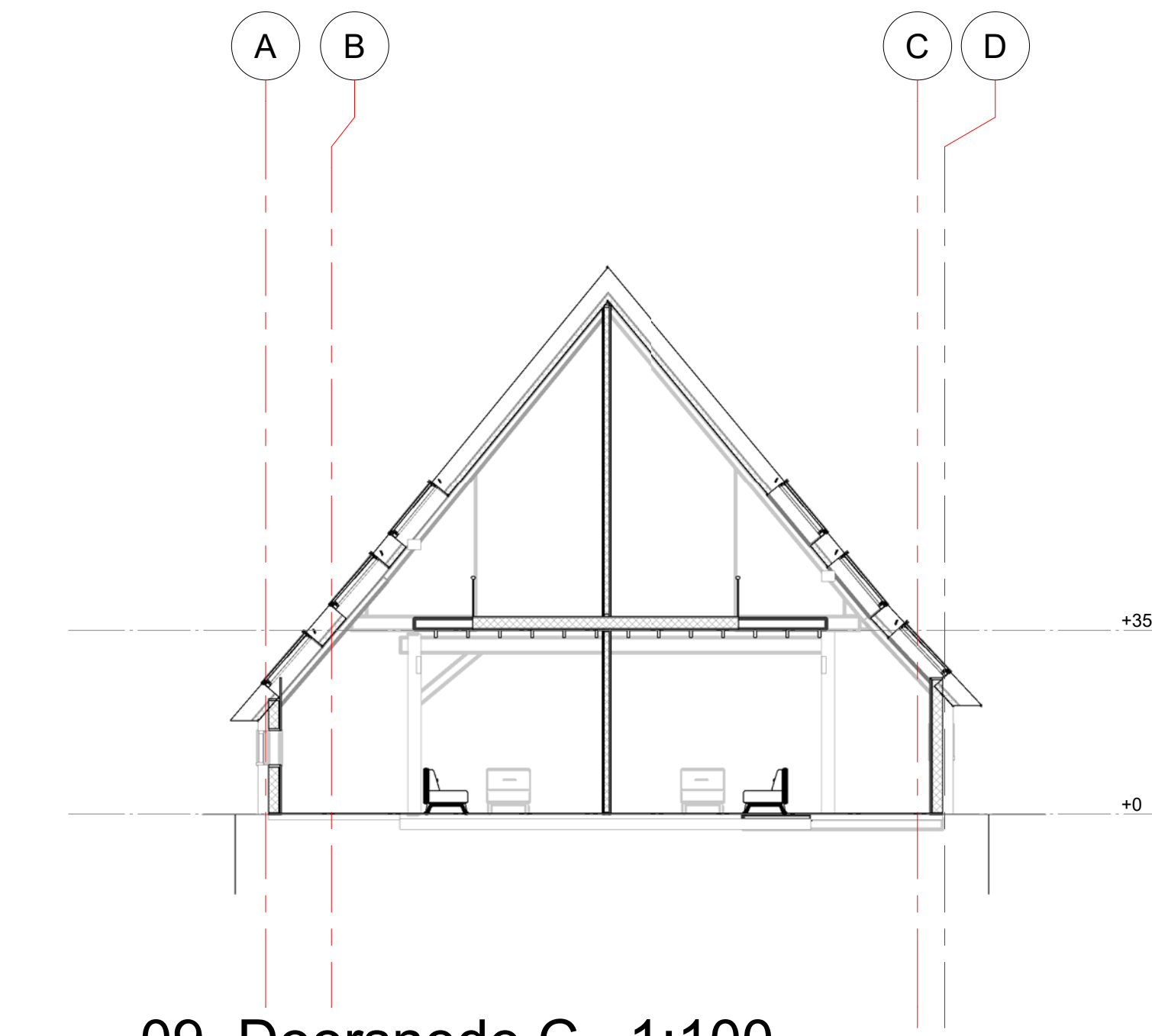
09. Doorsnede C 1:100
