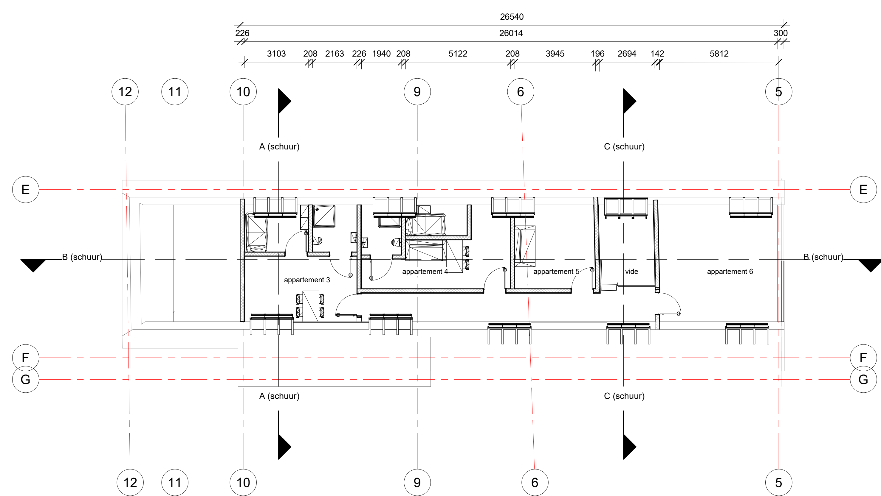
05. plattegrond BG 1:100
