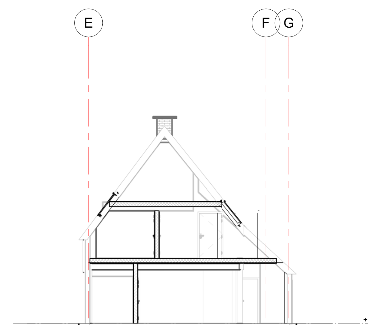
07. Doorsnede A 1:100
