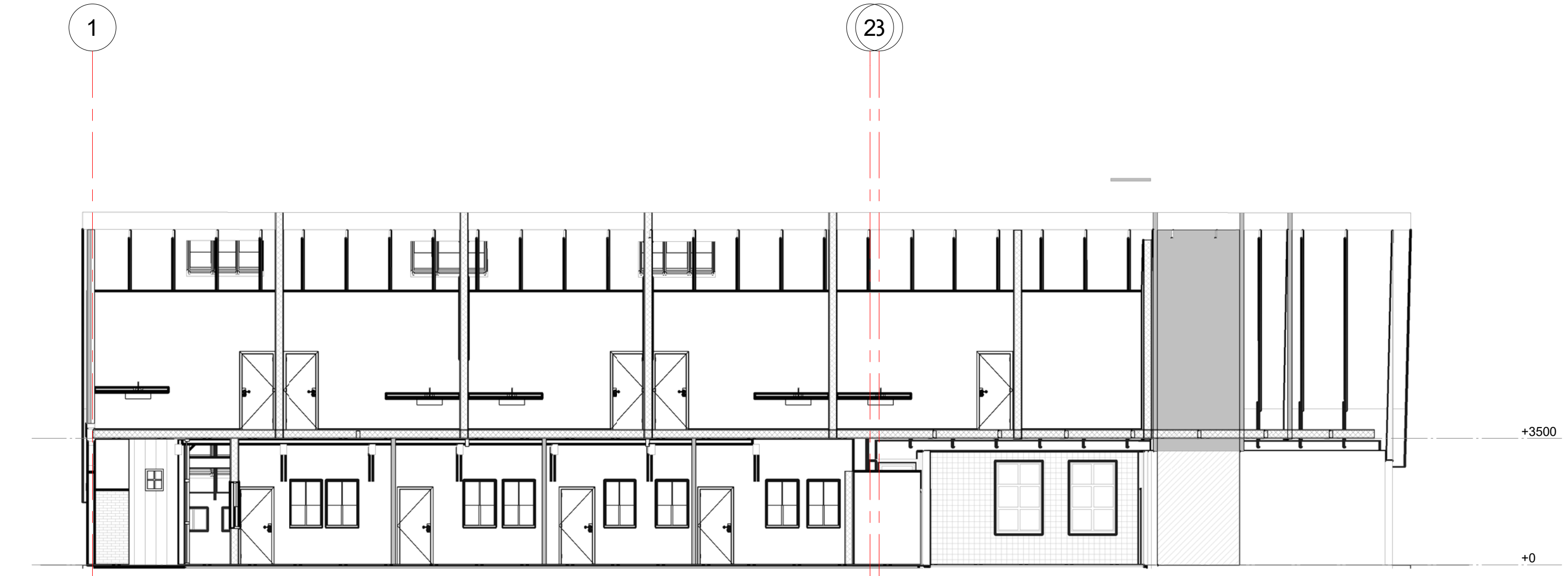
08. Doorsnede B 1:100
