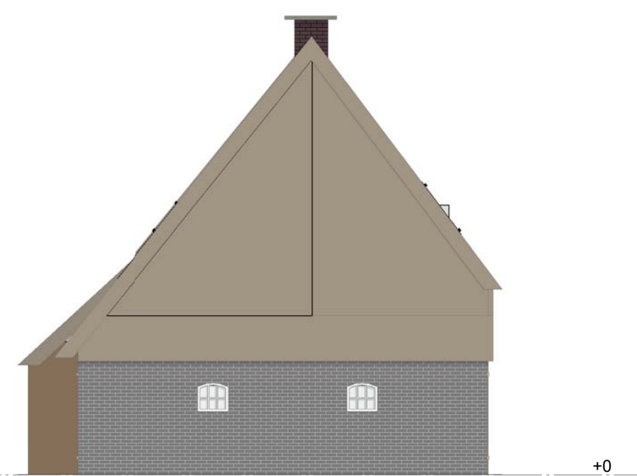
01. voorgevel 1:100
