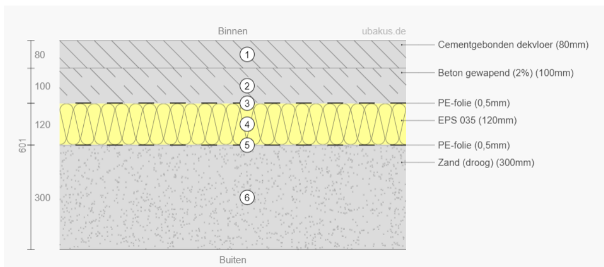
FIGUUR 17 OPBOUW BEGANE GRONDVLOER
