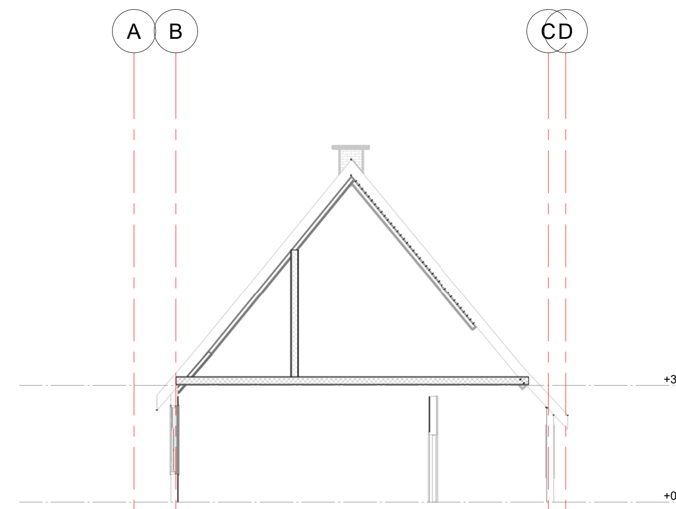
09. Doorsnede C 1:100
