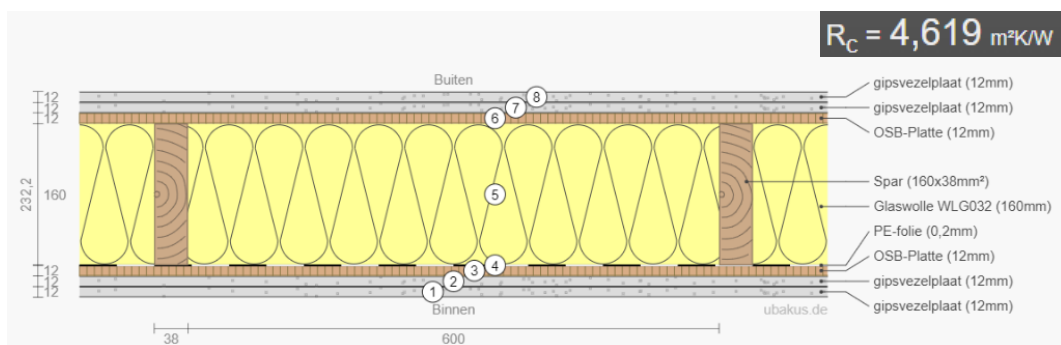
FIGUUR 34 - OPBOUW SCHEIDINGSWAND
