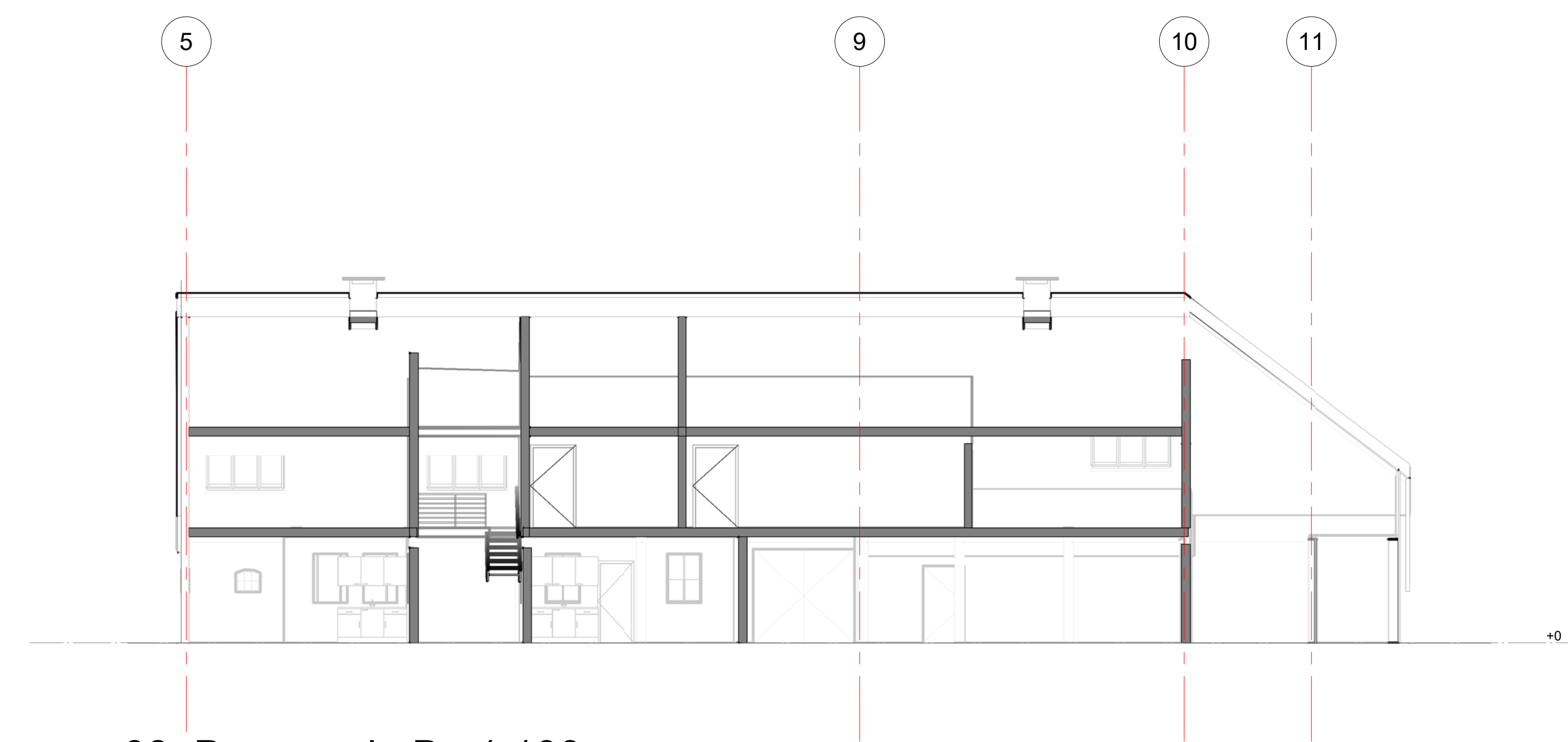
08. Doorsnede B 1:100
