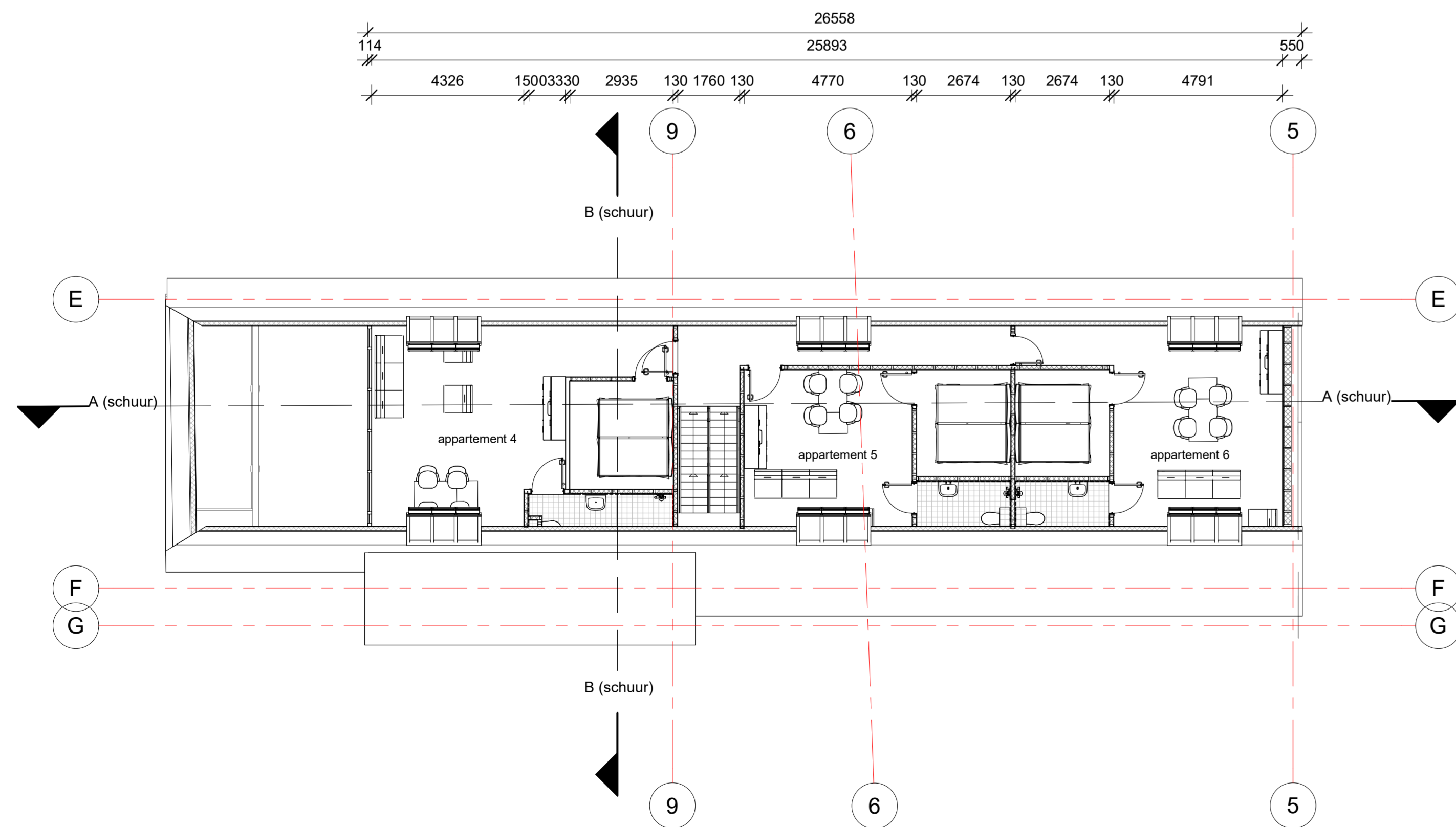
06. plattegrond V1 1:100
