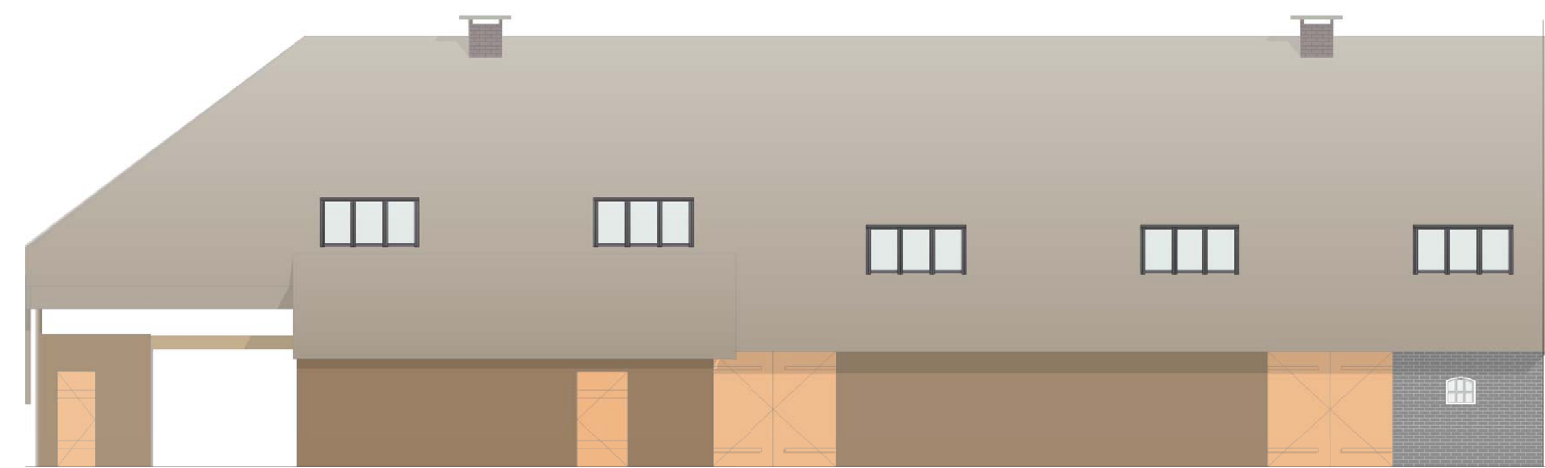
02. rechter zijgevel 1:100
