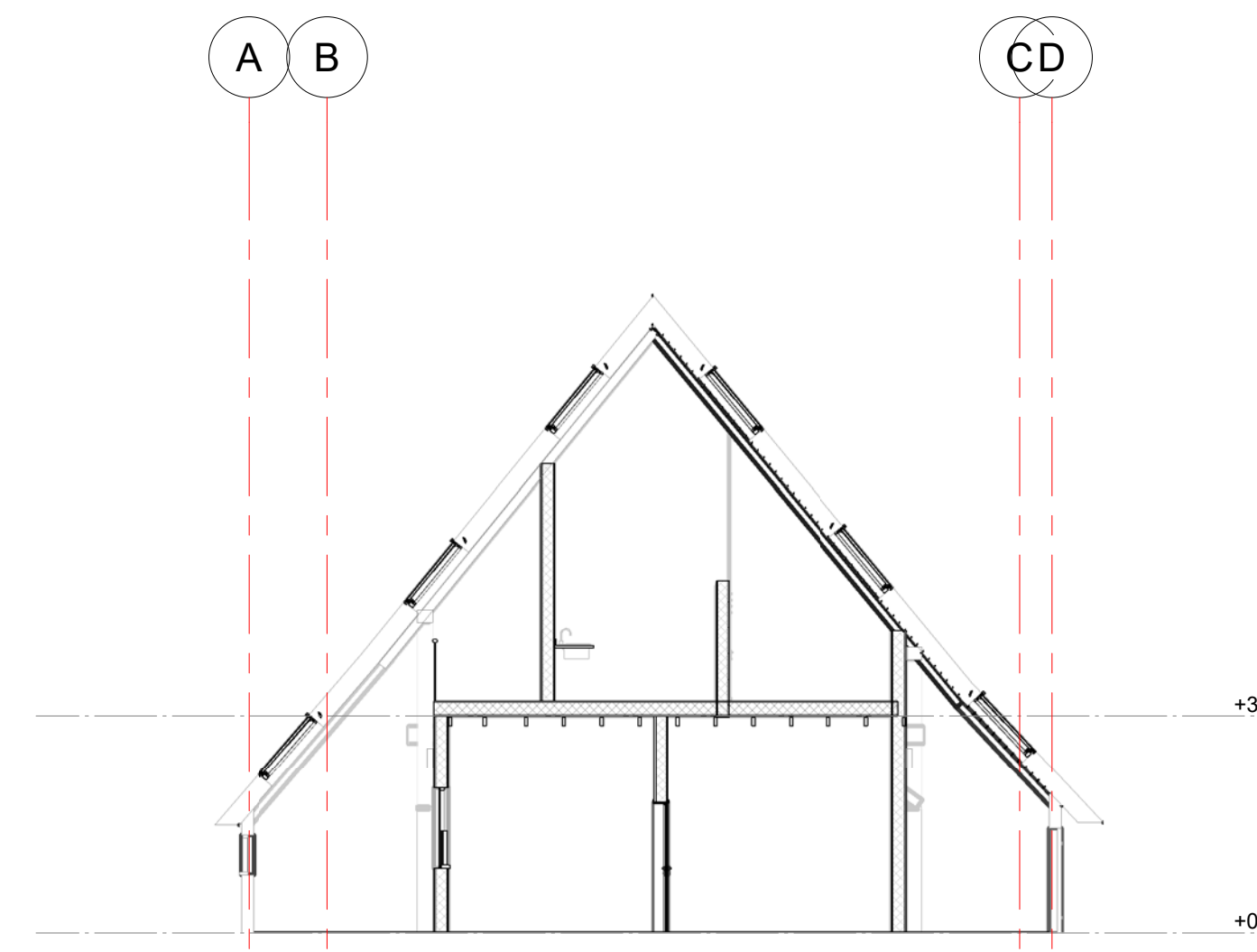
07. Doorsnede A 1:100
