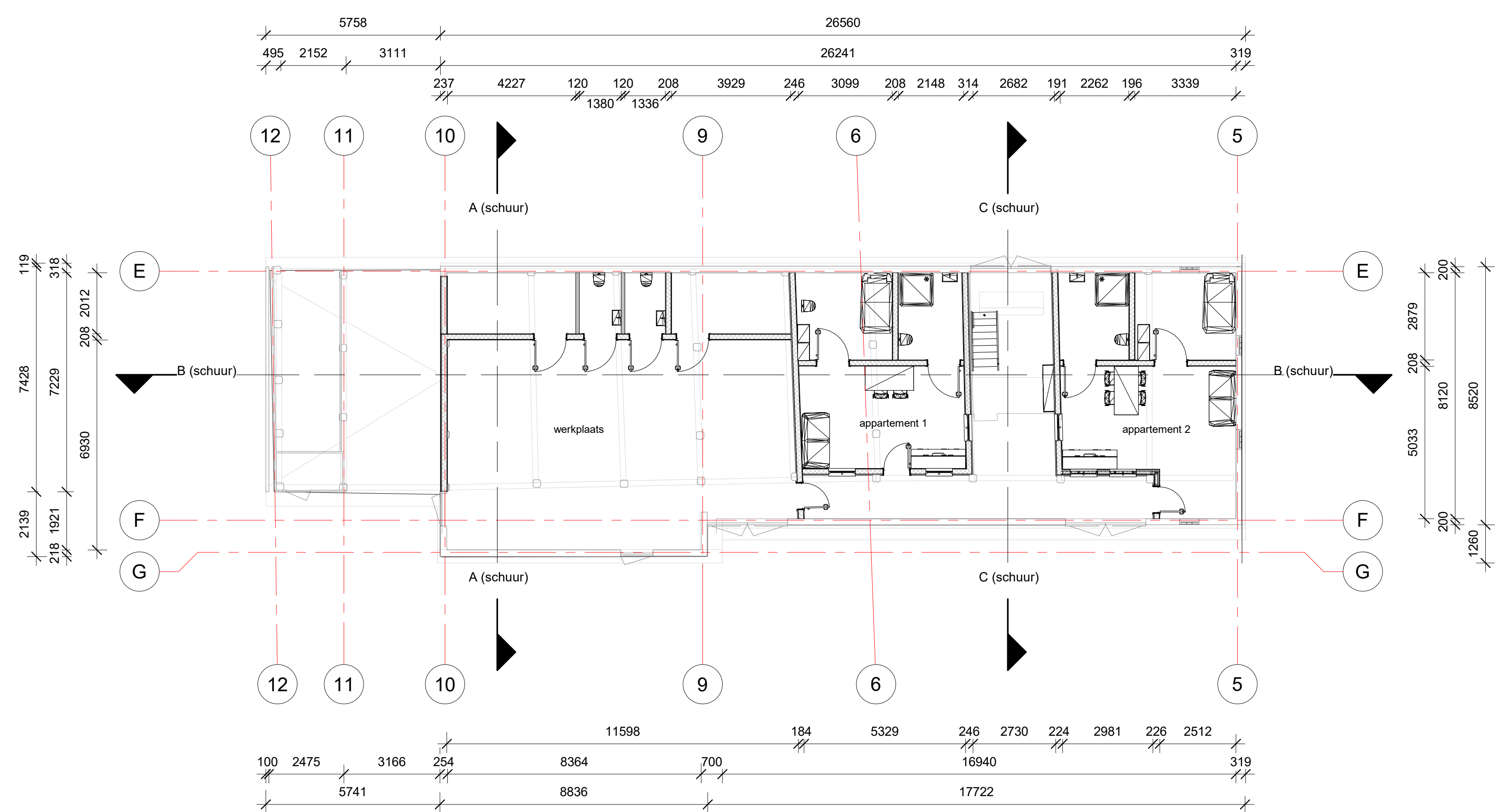
05. plattegrond BG 1:100
