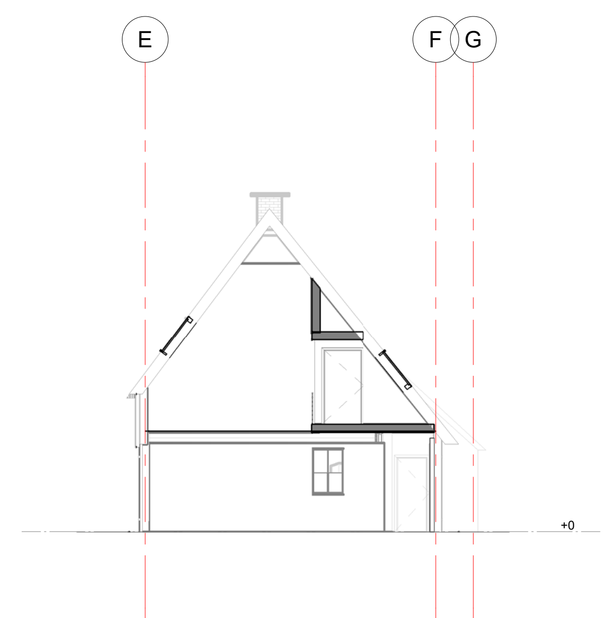
09. Doorsnede C 1:100
