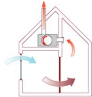
FIGUUR 24 -AFVOERMECHANISME
